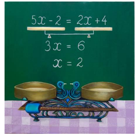
3. JEDNAČINA - TERAZIJE
