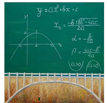
9. PARABOLA
