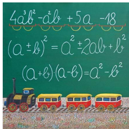
8. POLINOMI
